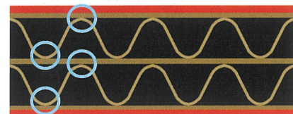
AA フルート (複両面段ボール)
