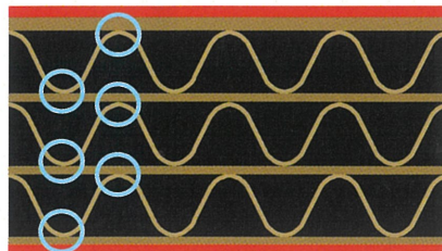
AAA フルート (複々両面段ボール)
